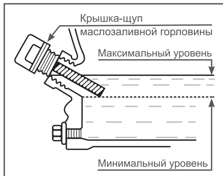
Рис. 12 Проверка уровня масла в картере 6. Плотнo закрутите крышку-щуп.
