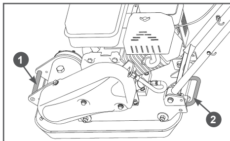
Рис. 36 Рукоятки транспортировочные
