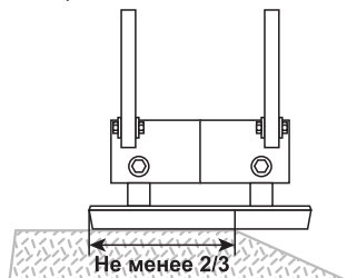
Рис. 12 Расположение виброплиты на краю обрабатываемой поверхности
