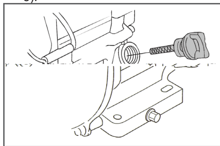
Рис. 5 Крышка-щуп маслосазливной горловины
